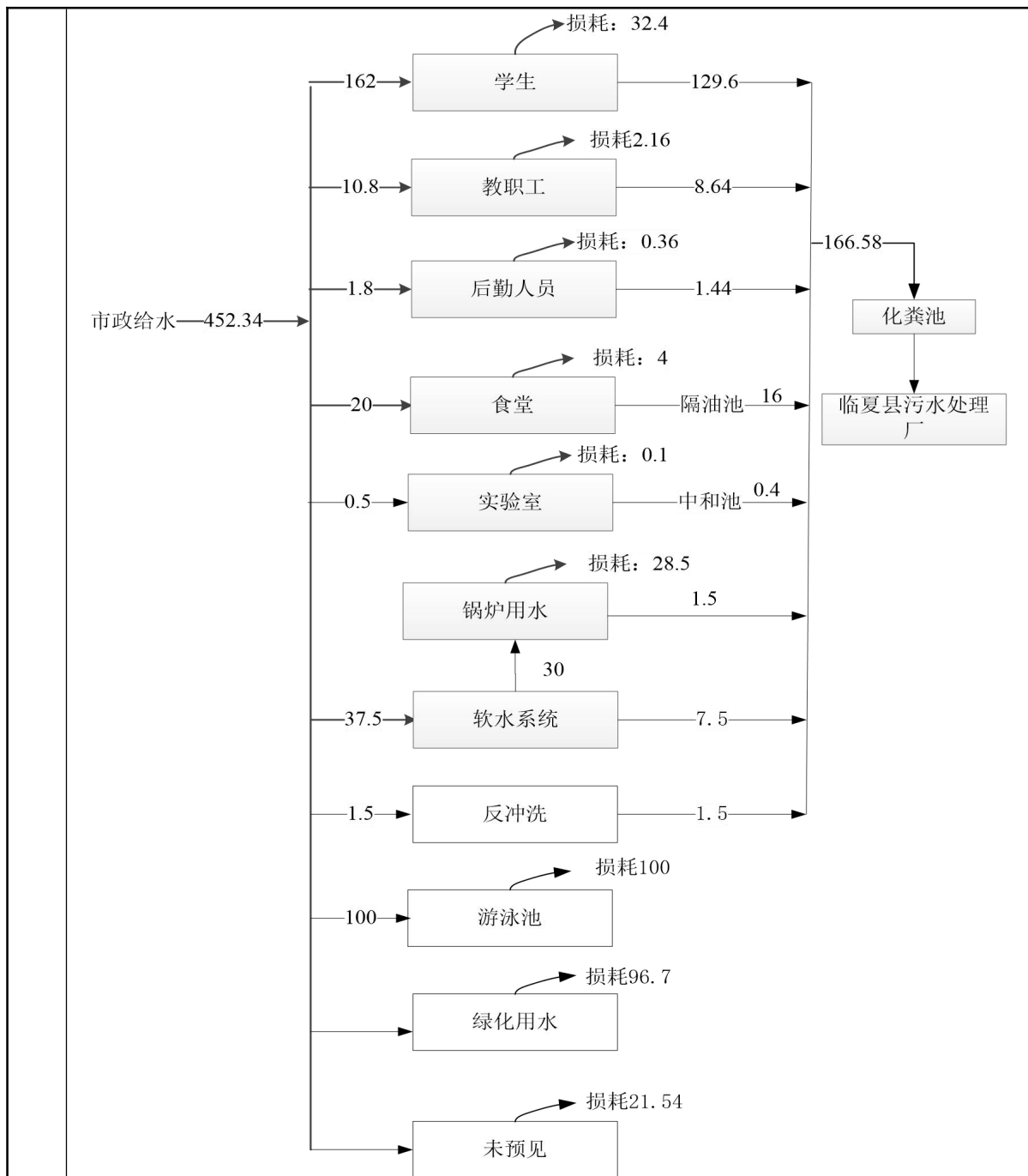
图 4 项目水平衡图 (单位: m³/d)
