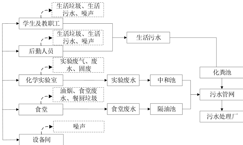
图 6 项目运营期工艺流程及污染流程图
